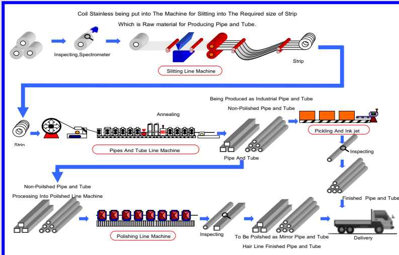
ภาพแสดงขบวนการผลิตท่อสแตนเลส
