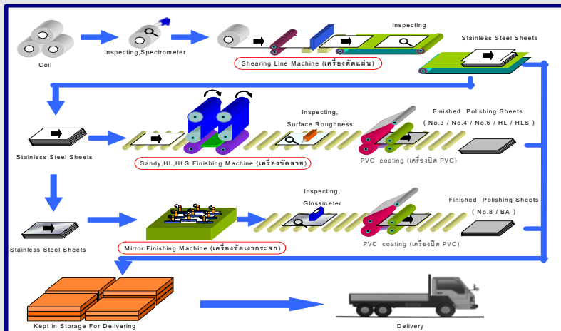
ภาพแสดงขบวนการผลิตแผ่นสแตนเลส
