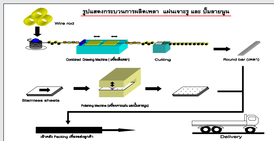
ภาพแสดงขบวนการผลิตแผ่นสแตนเลส
