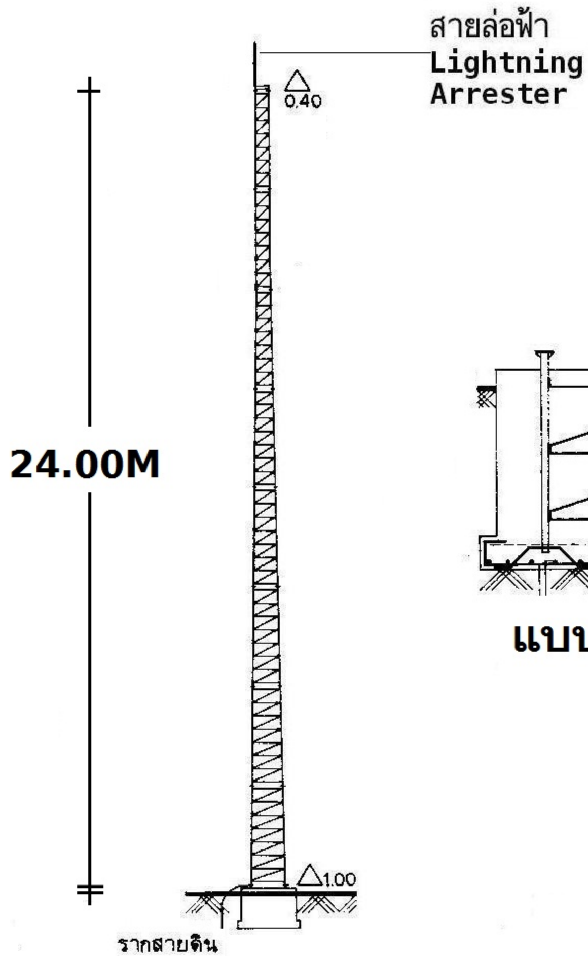
เสาโครงถักลอยตัว 24.00M SELF SUPPORT TOWER
