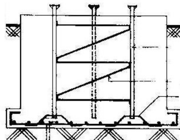
แบบฐานเสา
