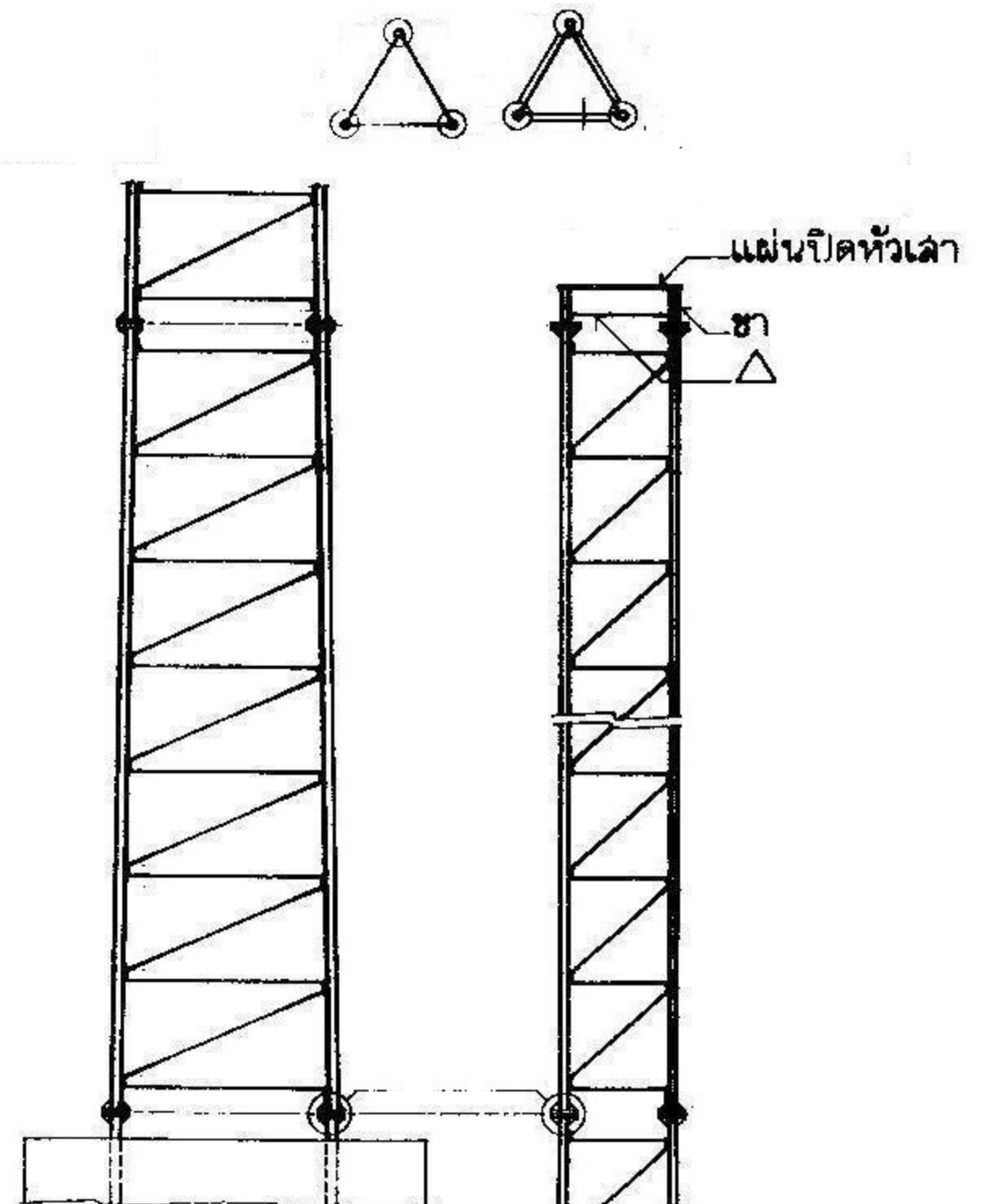
แบบเสา
