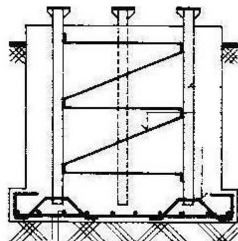
แบบขยายฐานเสา
