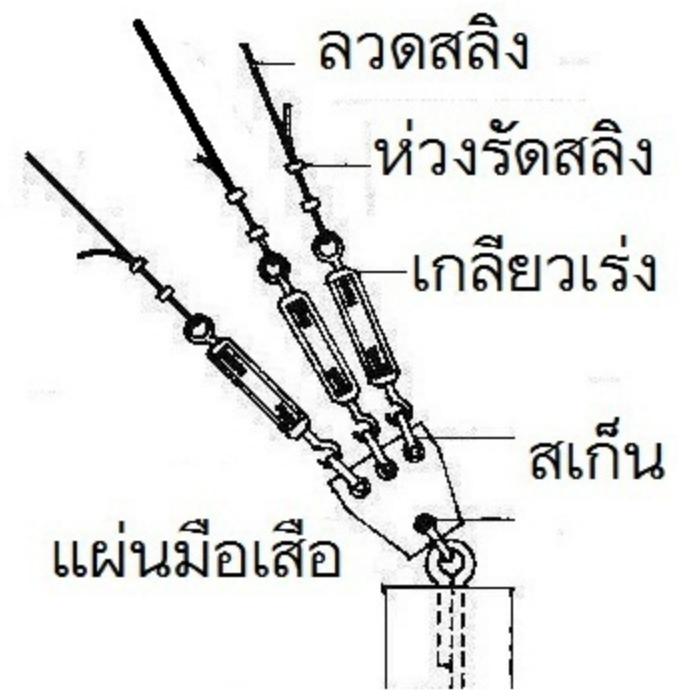
แบบแผ่นปรับลวดสลิง
