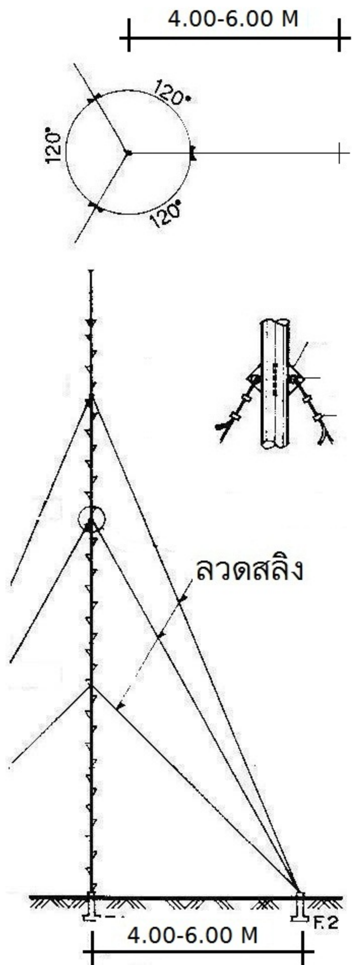
เสาเดี่ยวโยงลวดสลิง 18.00M GUYED - POLE
