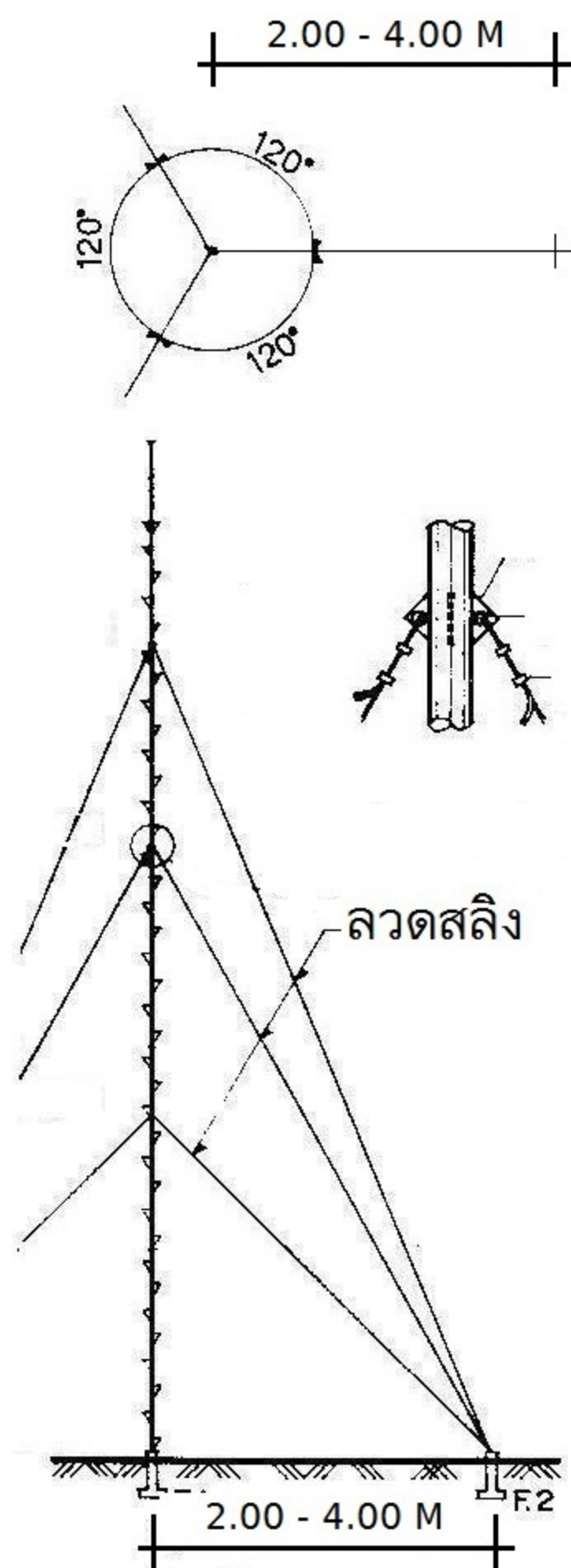
เสาเดี่ยวโยงลวดสลิง 15.00M GUYED - POLE
