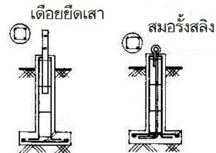
แบบขยายฐานเสา FOOTING DETAIL
