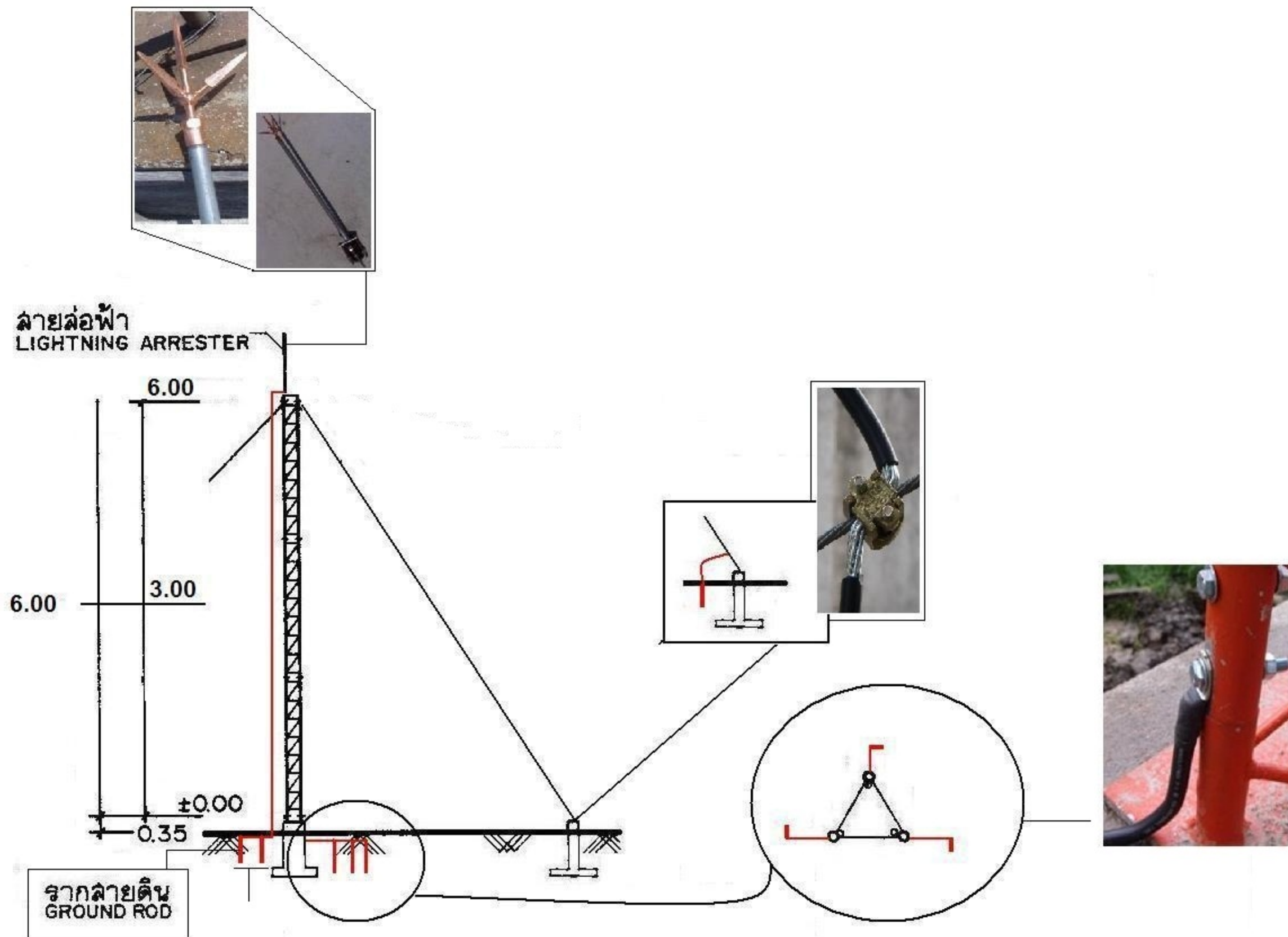
เสาคอนกรีตโยนลวดสลิง 6 M. GUYED-MAST TOWER
