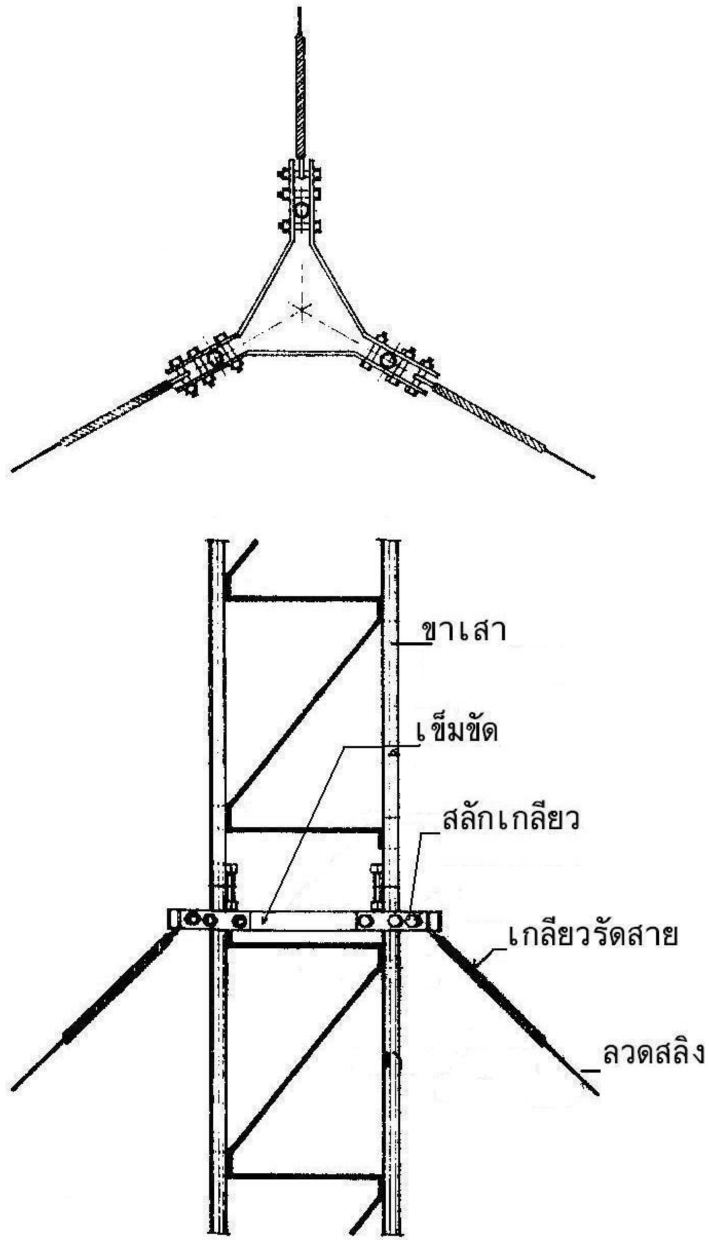
แบบขยาย เข็มขัด รัดสลิง
