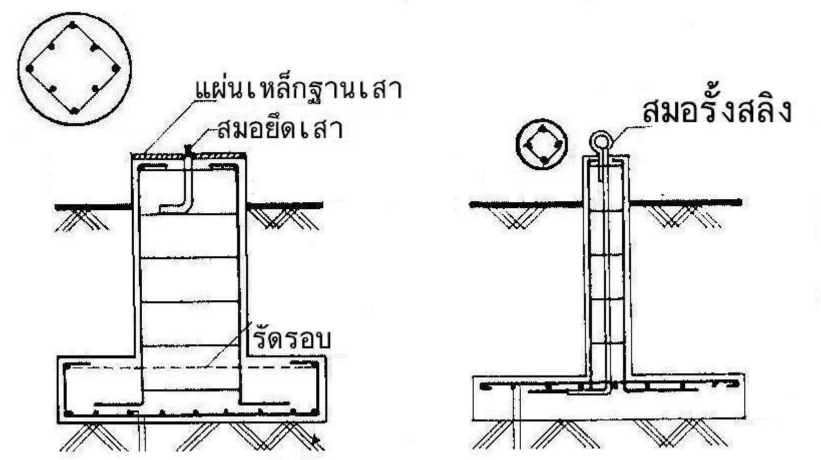
แบบขยายฐานเสา
