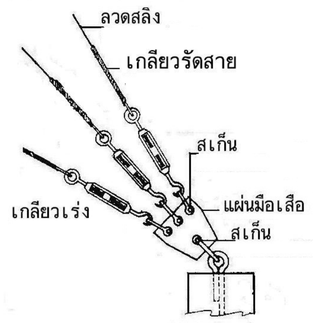
แบบแผ่นปรับลวดสลิง
